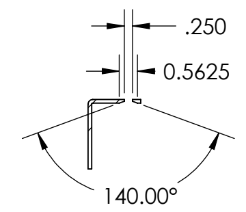
SECTION A-A SCALE 1 : 4
